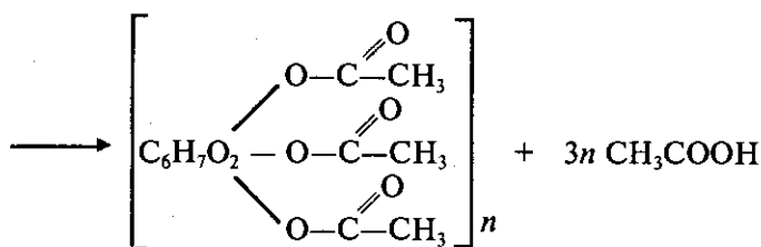
Триацетилцеллюлоза
