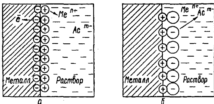
Рис. 23. Образование двойного электрического слоя на границе металл — раствор его соли \text{Me}_m\text{Ac}_n :
