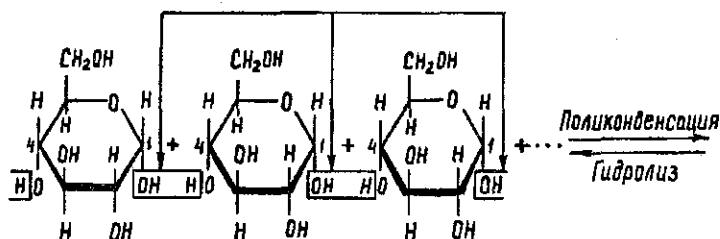
\alpha -Глюкоза
