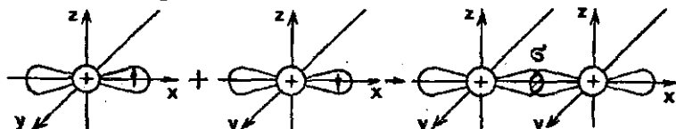
Рис. 4. Схема перекрывания электронных облаков в молекуле хлора
