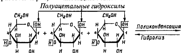
β-Глюкоза
