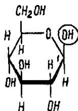
\beta -D-Глюкопираноза
