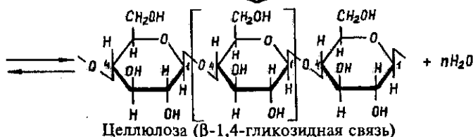
Структурное звено целлюлозы
