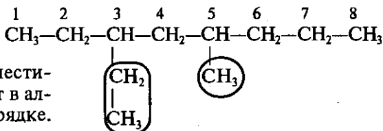
5-Метил-3-этилоктан
