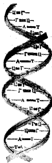
Рис. 37. Схематическое изображение двойной спирали ДНК (обозначения: S — остаток пентозы; P — остаток H_3PO_4 )
